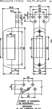
WERSJA MOCOWANIA 2 MOUNTING VERSION 2
