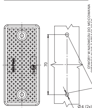
PIONOWA WERSJA MOCOWANIA VERTICAL MOUNTING VERSION
