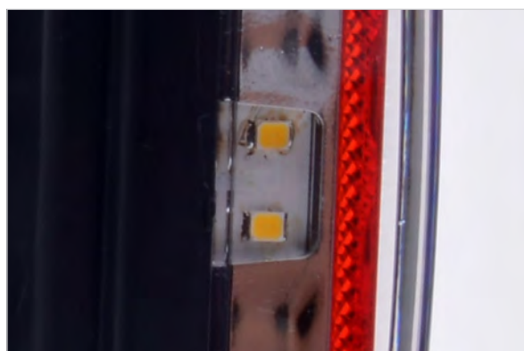
z bocznym oświetleniem tablicy / with license plate light on the side
