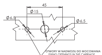
WIDOK WERSJI Z OZDOBNYM PIERSCIENIEM VIEW OF THE VERSION WITH DECORATING RING
