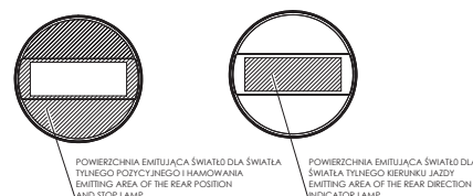
OGRANICZENIA W MONTAŻU LAMP JAKO ZESPÓŁ DWOCH ŚWIATEŁ NIEZALEŻNYCH RESTRICTIONS ON THE LAMP ASSEMBLY AS A SET OF TWO INDEPENDENT LAMPS
