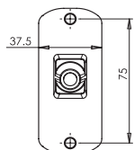
LAMPA Z WĄSKĄ PODSTAWĄ LAMP WITH NARROW BASE
