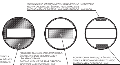
OGRODNIENIA W MONTAŻU LAMP JAKO ZESPÓŁ DWÓCH ŚWIATEŁ NIEZALEŻNYCH RESTRICTIONS ON THE LAMP ASSEMBLY AS A SET OF TWO INDEPENDENT LAMPS
