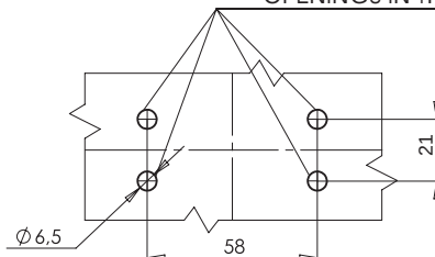
OTWORY W NADWOZIU DO MOCOWANIA OPENINGS IN THE CARRIAGE TO FIX
