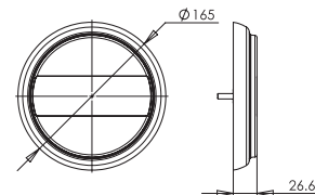
WIDOK WERSJI Z OZDOBNYM PIERSCIENIEM VIEW OF THE VERSION WITH DECORATING RING
